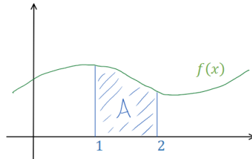
Abb. 15: Beispiel für Fläche unter dem Graphen von f(x) .
