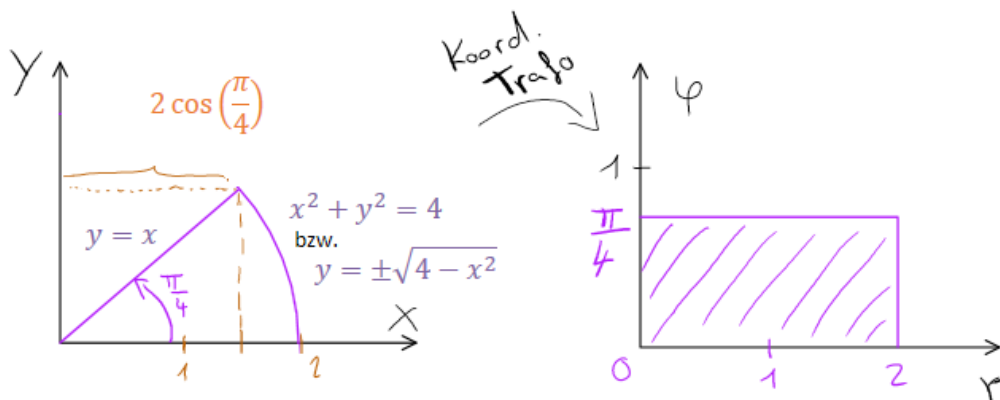
Abb. 19: Darstellung des Integrationsbereichs in kartesischen (links) und polaren Koordinaten (rechts).
