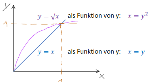
Abb. 18: Darstellung der Situation im Beispiel: Integrationsbereich mit variablen Grenzen bzgl. y .
