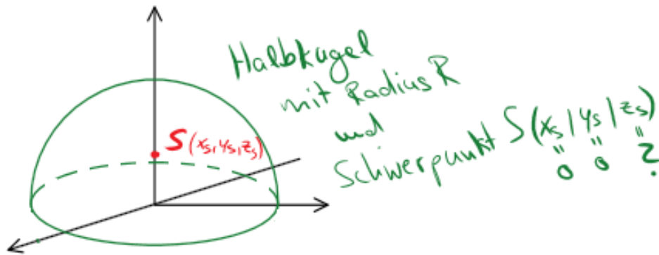
Abb. 26: Darstellung des Schwerpunktes der homogenen Halbkugel.
