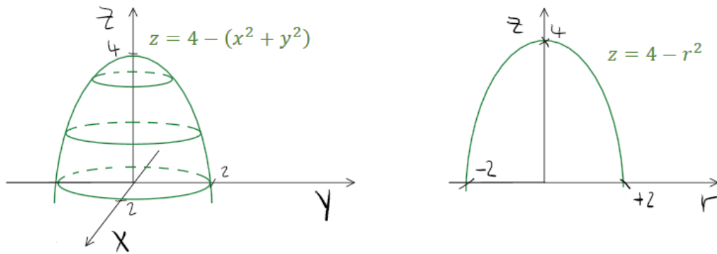
Abb. 21: Darstellung des Integrationsbereichs in kartesischen (links) und polaren Koordinaten (rechts).
