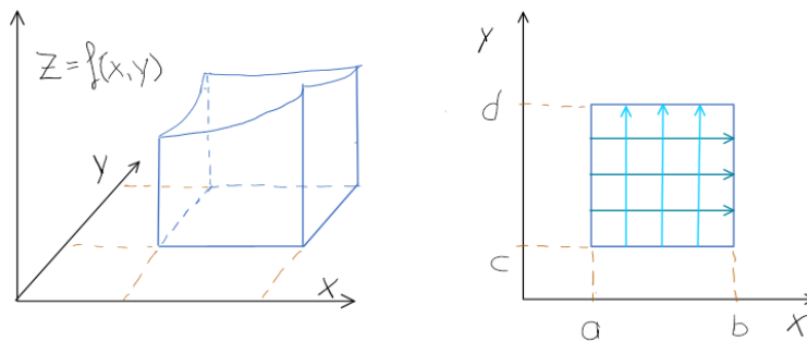
Abb. 16: Beispiel für Volumen unter dem Graphen eines Skalarfeld z = f(x, y) .
