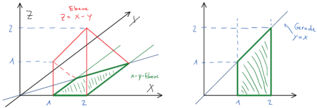
Abb. 23: LINKS: Darstellung des dreidimensionalen Integrationsbereichs des Beispiels (Papula, Band 2, Seite 306). RECHTS: Darstellung der grünen Grundfläche in der x - y -Ebene.
