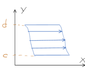
Abb. 17: Darstellung eines Integrationsbereichs mit variablen Grenzen bzgl. x .
